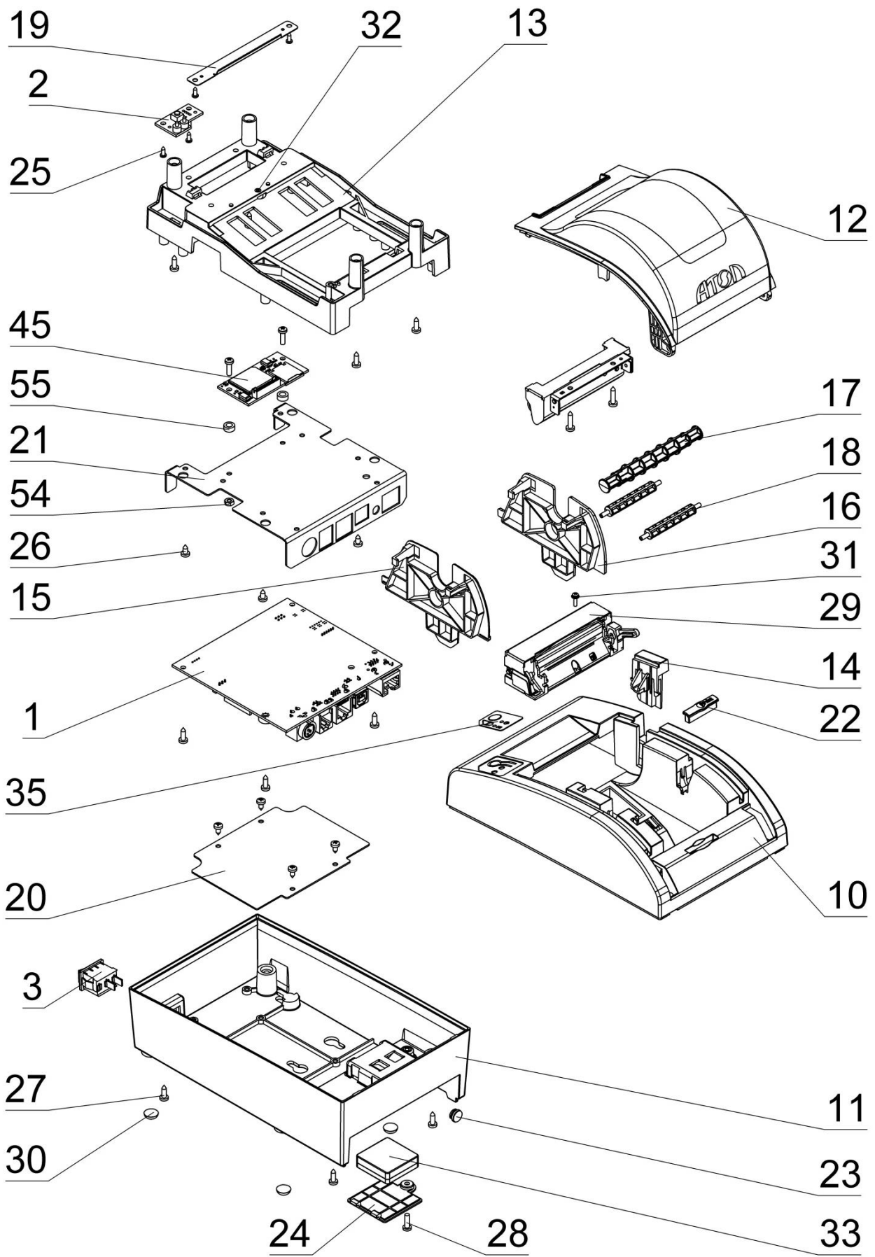
Рисунок 1. Компоновочная схема ККТ АТОЛ 55Ф
